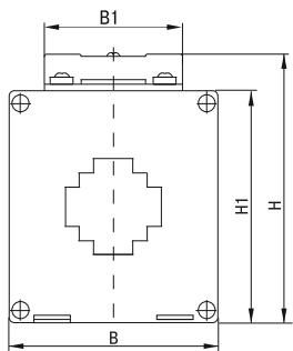
б) модификации ТТИ-30 габарит 2
