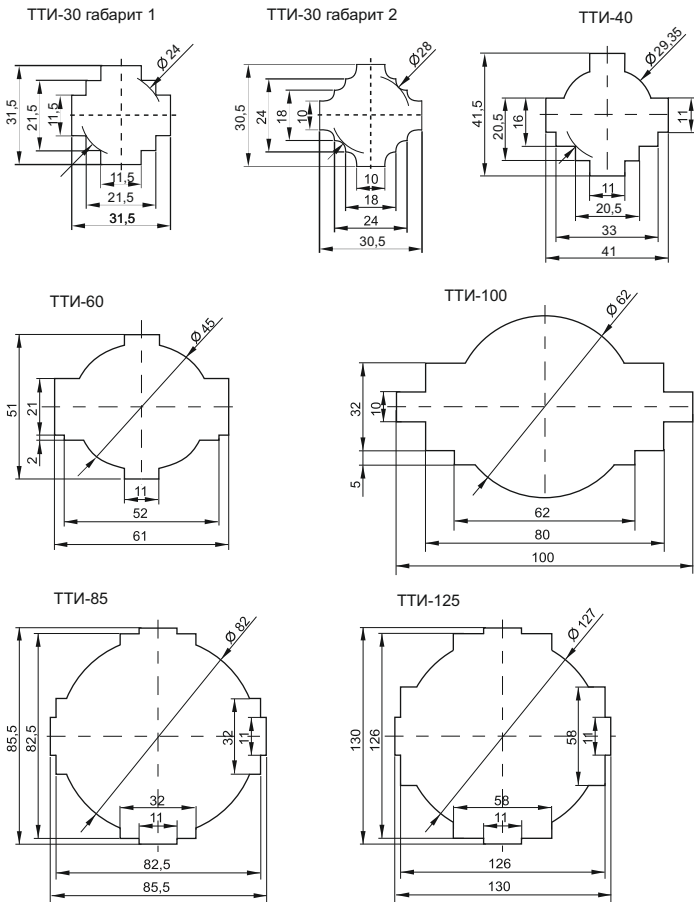
Рисунок 3 – Размеры отверстий под шины и кабели
