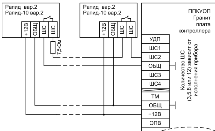
Рис.Б4 Схема подключения охранных извещателей Rapid вар.2, Rapid-10 вар.2
