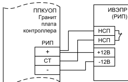
Рис.Б6 Схема подключения источника внешнего электропитания резервированного (РИП)
