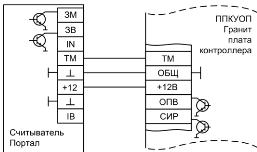
Рис.Б5 Схема подключения считывателя «Портал»
