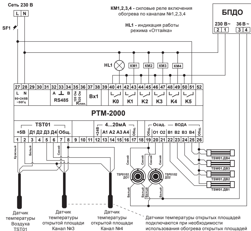
Рис. 21. Типовая схема включения алгоритма «КРОВЛЯ/ДОР».
