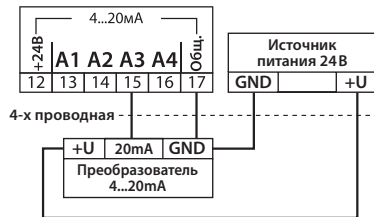
Рис. 18. Схемы подключения преобразователей в унифицированный сигнал 4...20 мА
