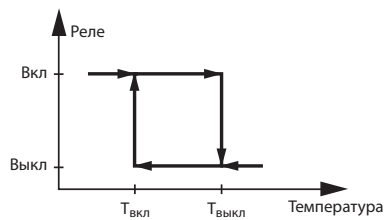
Рис. 10. Гистерезис работы.
