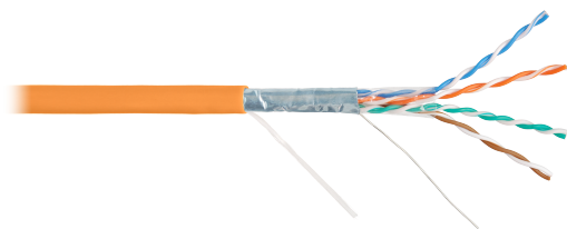
Кабель NIKOLAN F/UTP, 4 пары, Кат.5е, 24 AWG, внутренний, LSZH, 305м/100м, где xx-цвет
