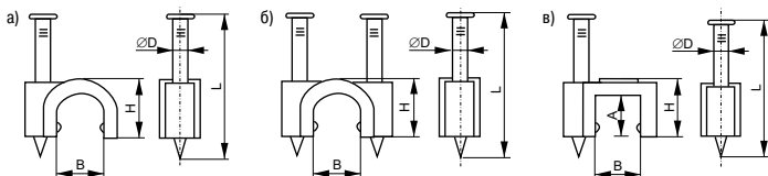
Рис.1 Габаритные размеры скоб: а) СКК4 ...СКК25; б) СКК30, СКК35; в) СКП
