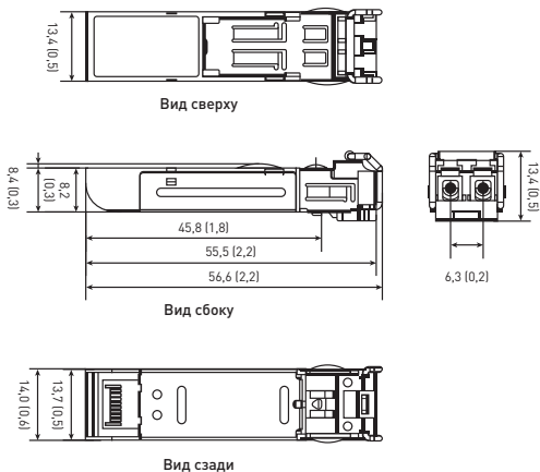
Рис. 1 — Габаритные размеры TSX-SFP-GS2D-13-20
