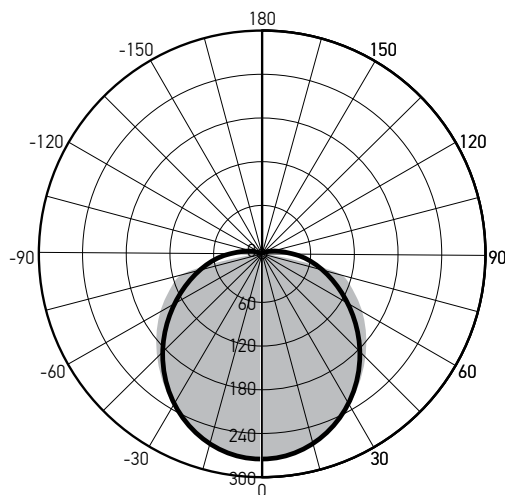
Светораспределение светильника PBH-PC2-RS 12W 960Lm 4000K
