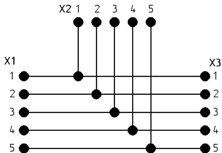
Принципиальная схема
