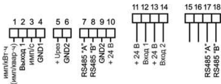
Схема подключения НЕВА СТ4ХХ с дополнительным модулем IO20E4
