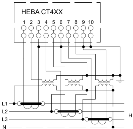
Схема включения счетчика HEBA CT4XX через трансформаторы тока и трансформаторы напряжения в четырехпроводную сеть
