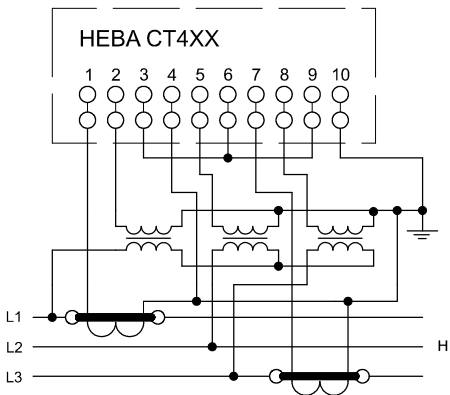
Схема включения счетчика НЕВА СТ4ХХ через два трансформатора тока и три трансформатора напряжения в трехпроводную сеть
