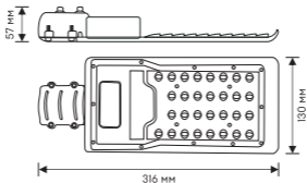
Рис. 1 - Габаритные размеры светильника ДКУ-9001-Ш
