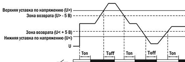
Рис. 3. Контроль напряжения
