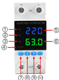
Рис. 2. Индикация и органы управления
