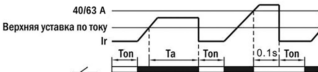
Рис. 4. Контроль силы тока
