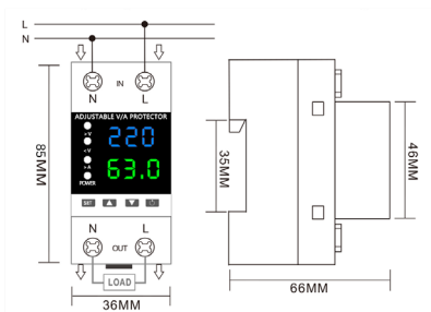
Рис. 1. Схема подключения и габаритные размеры
