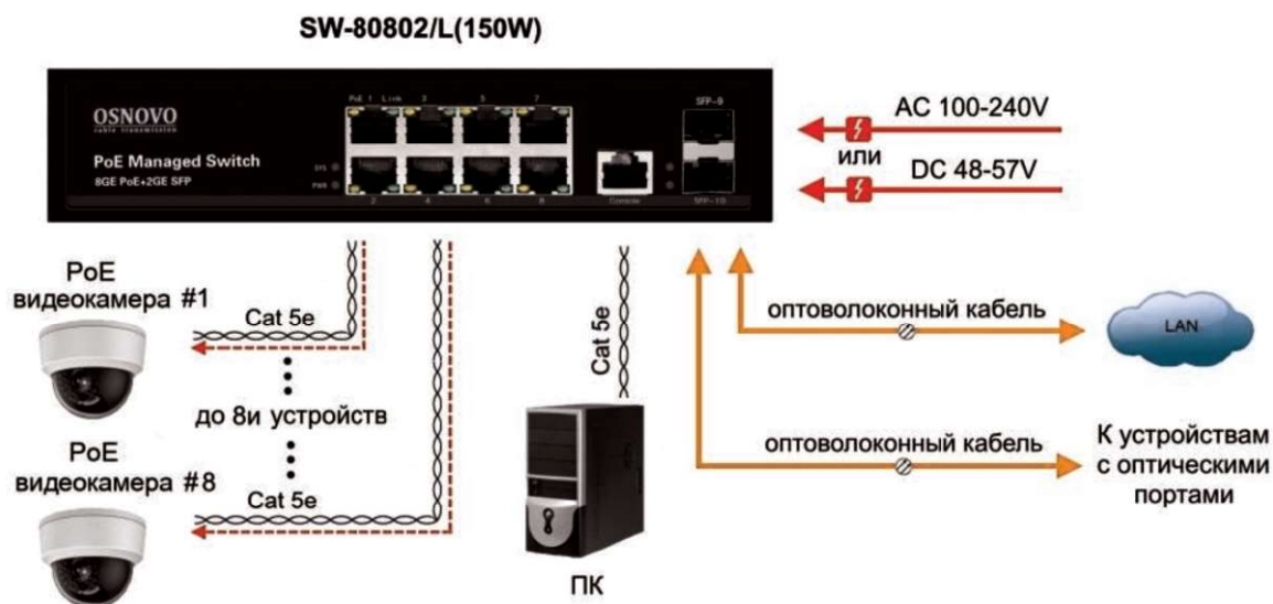
Рис.3 Типовая схема подключения коммутатора SW-80802/L(150W)
