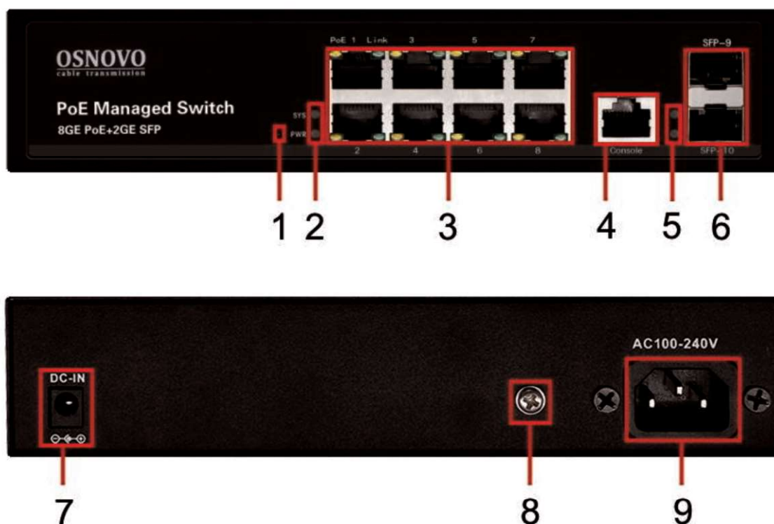
Рис.2 Панели подключения коммутатора SW-80802/L(150W)
