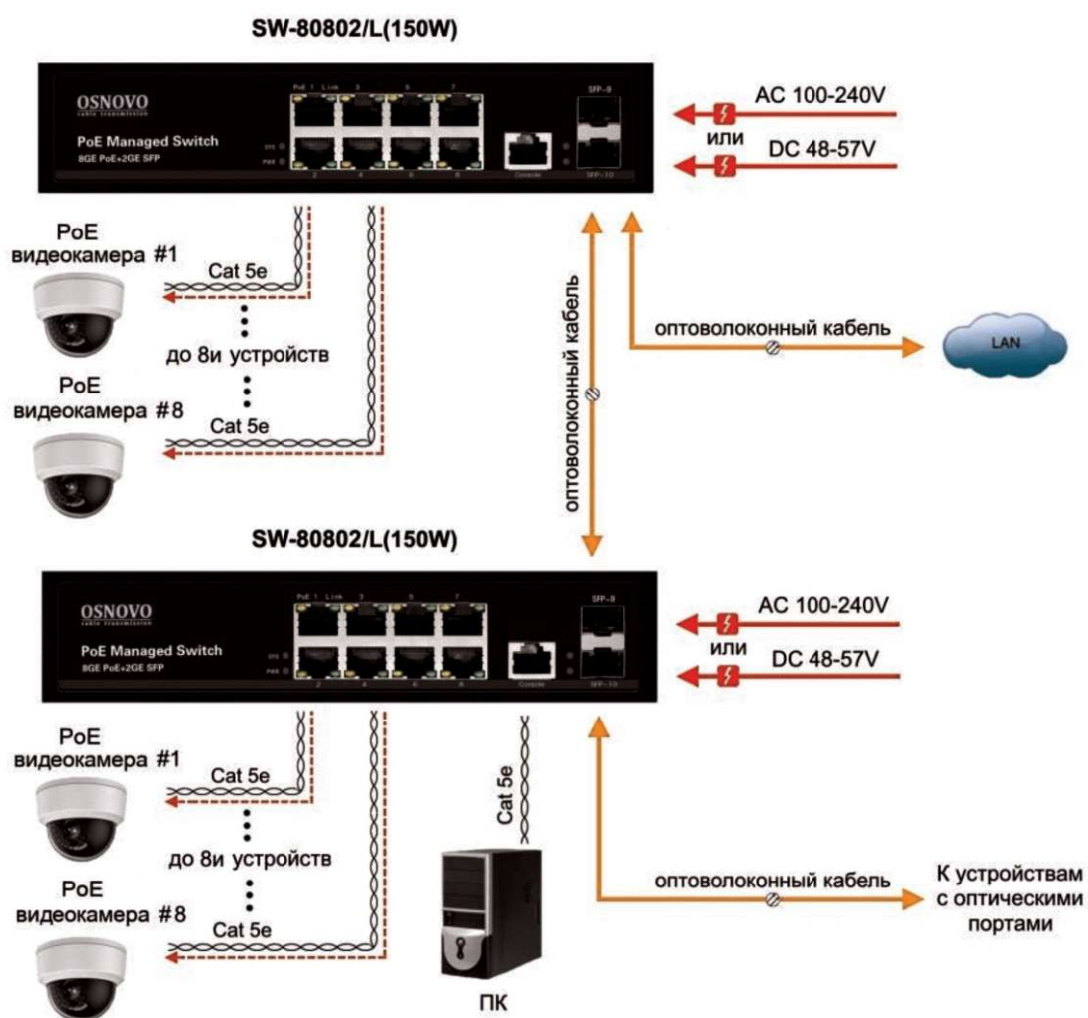
Рис.4 Схема каскадного подключения коммутатора SW-80802/L(150W)
