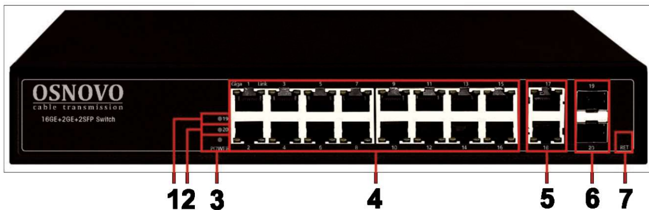
Рис. 3 Коммутатор SW-8182/L(300W), разъемы и индикаторы на передней панели
