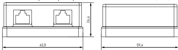
Рис. 2 Габаритные размеры TRC-WBOX-2RJ45-5EUTP-WH (в мм)
