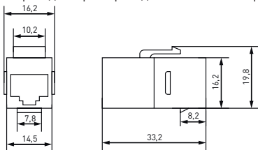
Рис. 3 Габаритные размеры TRC-INLC-KSTN-5EUTP-WH, TRC-INLC-KSTN-5EFTP (в мм)
