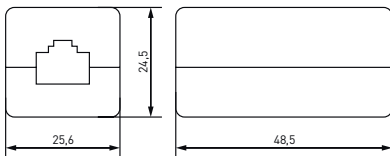
Рис. 4 Габаритные размеры TRC-INLC-2RJ45-5EUTP-WH (в мм)
